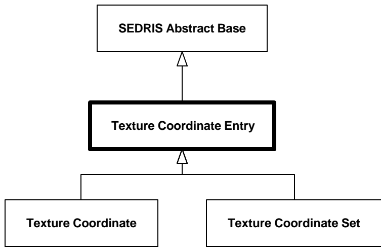
Diagram 6.289--DRM_Texture_Coordinate_Entry
