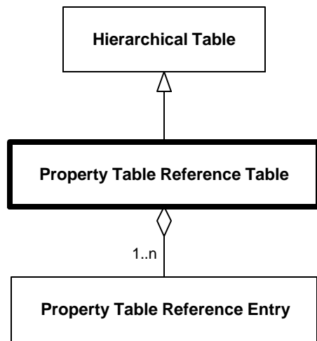
Diagram 6.218--DRM_Property_Table_Reference_Table
