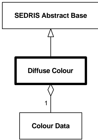
Diagram 6.73—DRM_Diffuse_Colour
