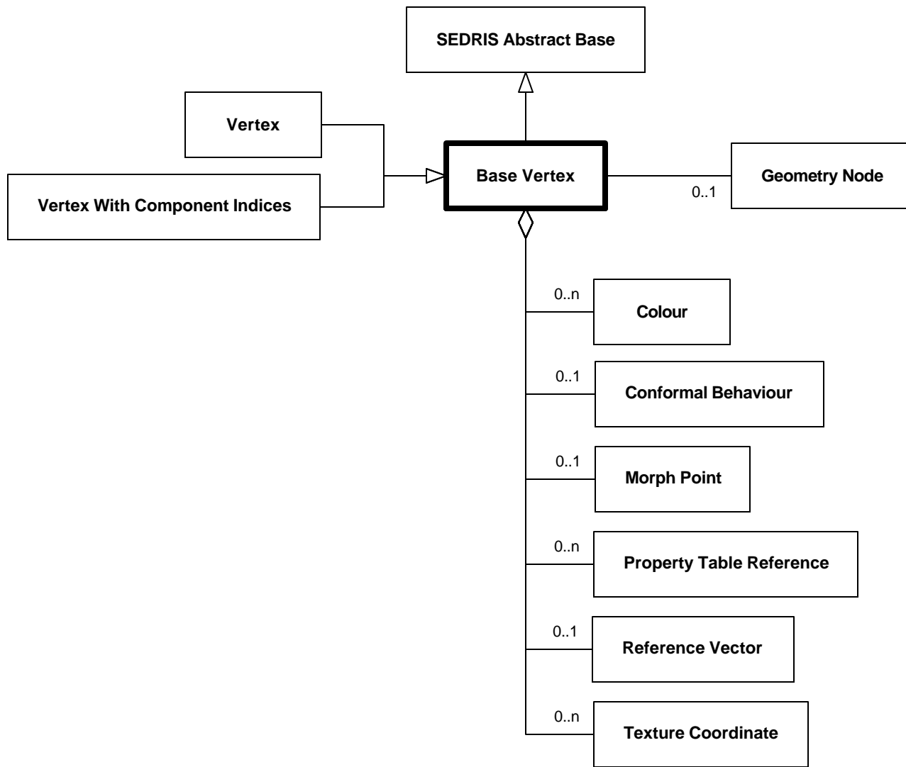
Diagram 6.34--DRM_Base_Vertex
